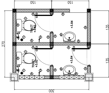
DETAIL TOILET A LI.2 SKALA 1 : 50
