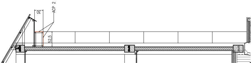
POTONGAN 5 FASAD SKALA 1 : 50
