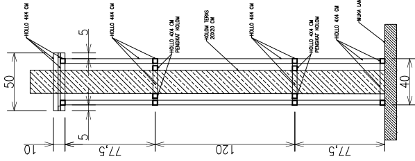
POTONGAN 6 FASAD
