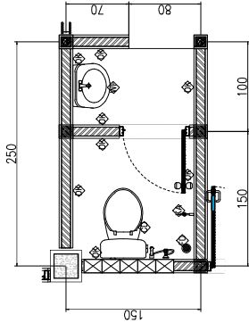
DETAIL TOILET A LI.1 SKALA 1 : 50
