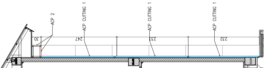
POTONGAN 4 FASAD SKALA 1 : 50
