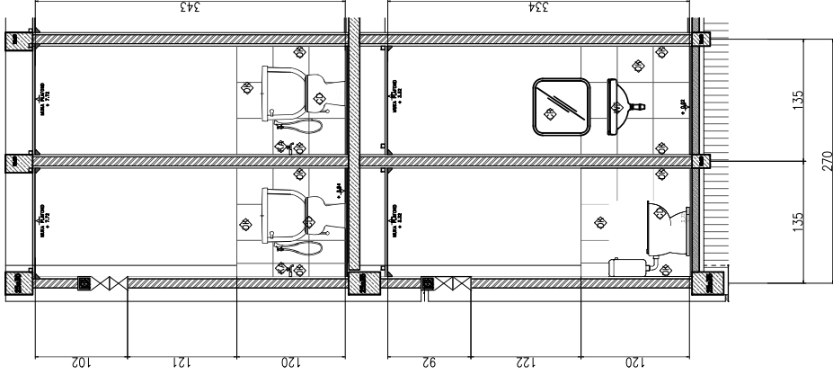
POTONGAN 1 SKALA 1 : 50
